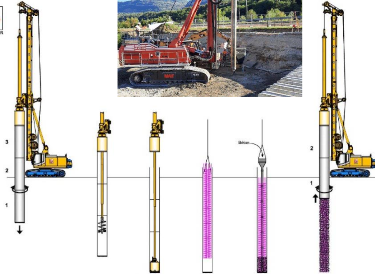
Mise en place de la colonne de tubes, constituée d'éléments vissés, par forage et rotation
