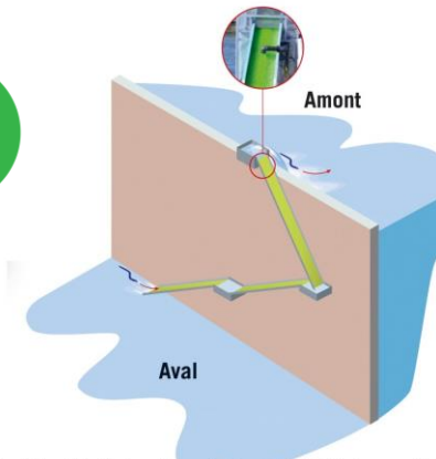
Pour l'Anguille, l'usine-écluse de Beaucaire Vallabrègues a été équipée de deux rampe de reptation avec brosses "ever green" parcouru par une lame d'eau permettant le franchissement de l'obstacle. La passe utilise la faculté de migration par reptation des anguilles.
